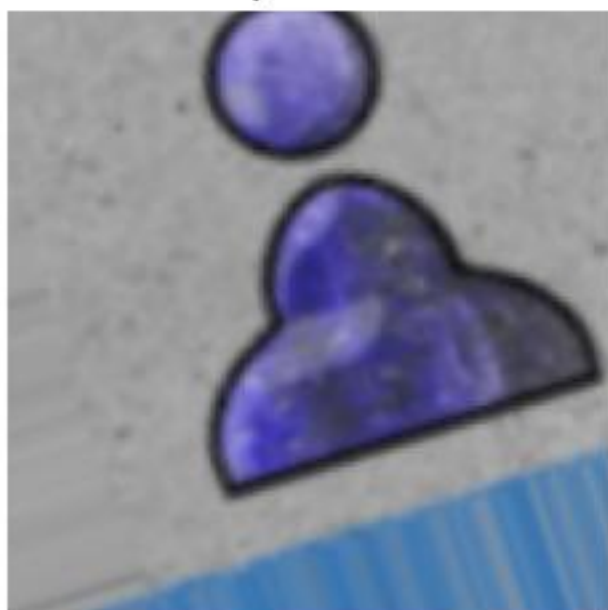
pawn
