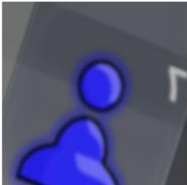
pawn
